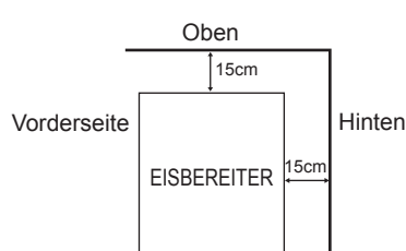
Seitenansicht
