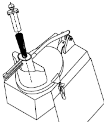
Рис. № 27 – Загрузка продукта через направляющий желоб на рычаге
