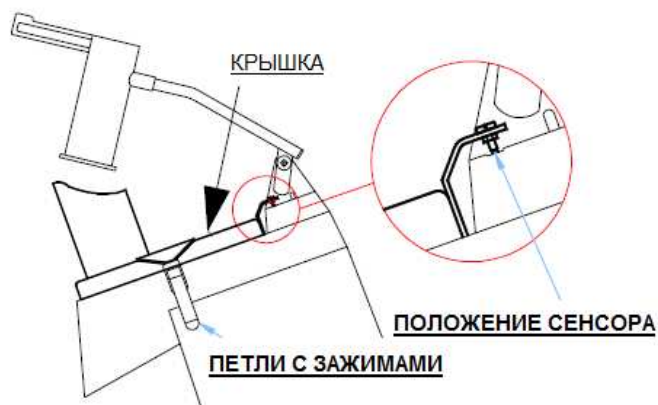
Рис. №3 – Устройство для механической безопасности
