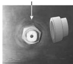
Кнопка Reset
