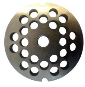
Решітка MEM 12 (8) Матеріал: нержавіюча сталь Ø отворів: 8 мм Машини: MEM 12
