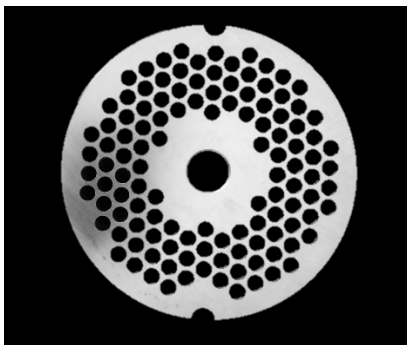
Решітка MEM 22 (4,5) Матеріал: нержавіюча сталь Ø отворів: 4,5 мм Машини: MEM 12
