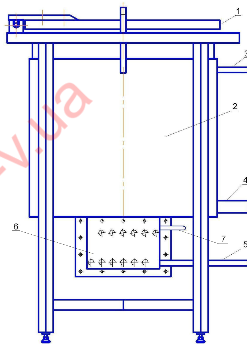
1- кришка, 2 - емність, 3- вхідна труба для проточної води, 4 - труба зливу продукту, 5 - вихідна труба для проточної води, 6 - парогенератор, 7 - пробно-спусковий кран
