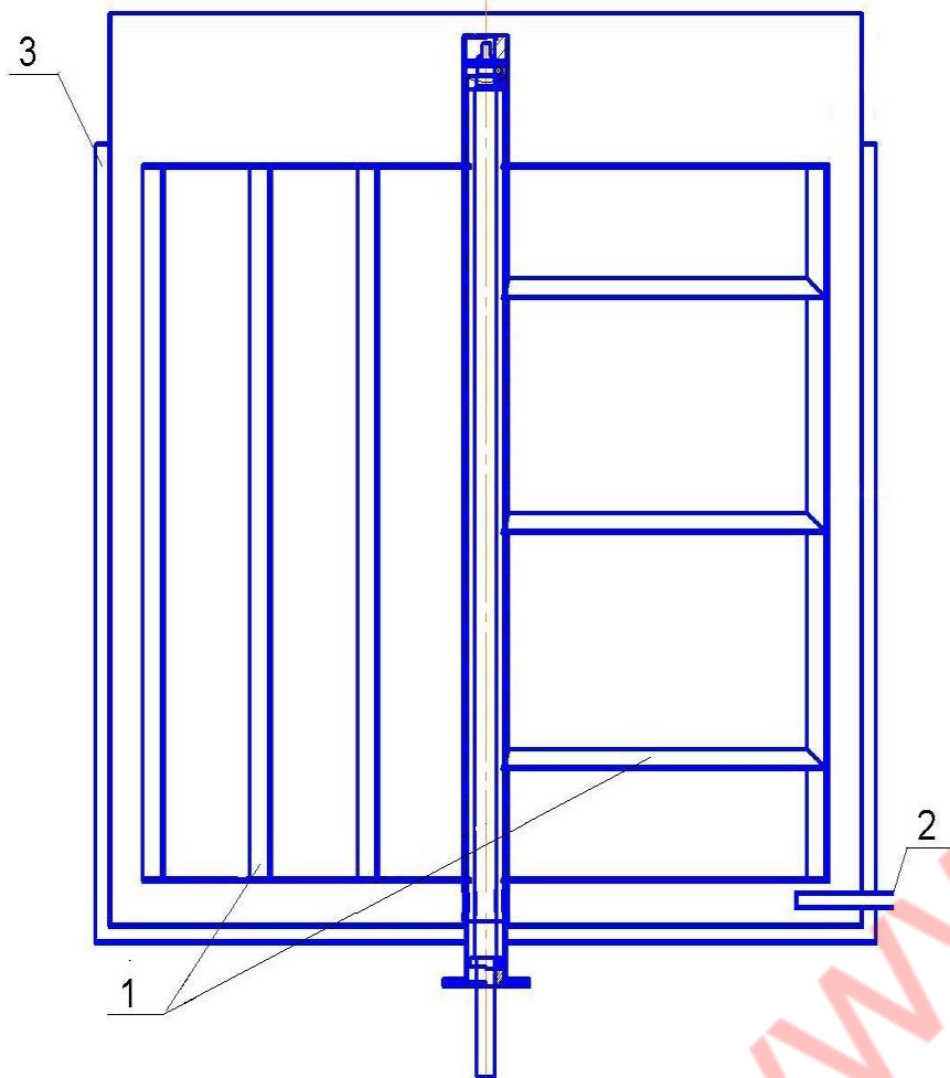
1 - перемішувач, 2 - труба для датчика, 3 - сорочка котла
