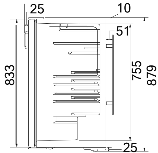
ВИД СБОКУ
