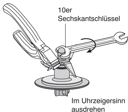
Abnehmen des Messers
