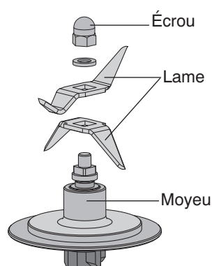
Éléments bloc-couteau
