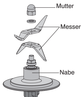
Messerblockelemente
