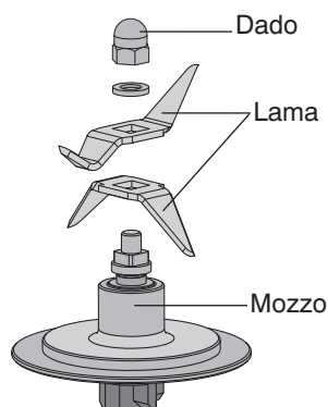
Elementi blocco lama
