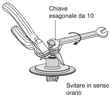
Smontaggio lama
