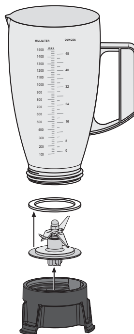
Entfernen des Messerblocks
