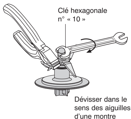
Démontage couteau
