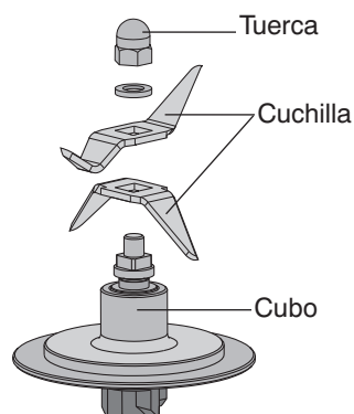
Elementos bloque cuchilla
