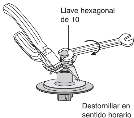
Desmontaje cuchilla
